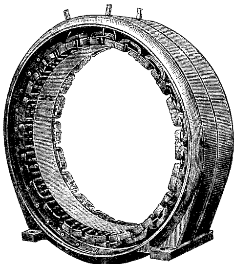
Статоръ тихоходнаго двухфазнаго двигателя Броуна.
