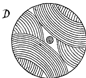
Двухполюсное поле Тесла декабрь 1889.
