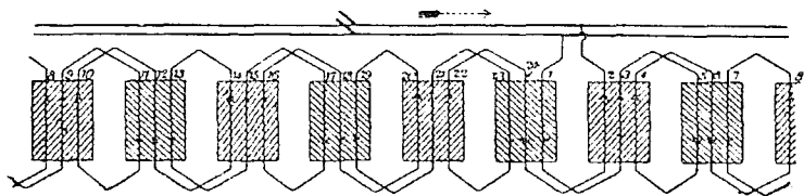
Машина переменнаго тока: петлеобразная обмотка.
