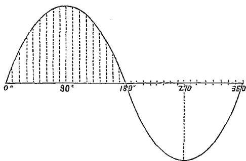
Кривая индуцированной электродвижущей въ обыкновенномъ (однофазномъ) альтернаторѣ.
