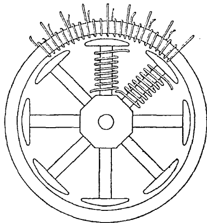
Альтернаторъ Грамма.
