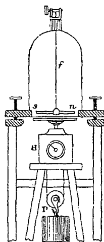
Вращающийся дискъ Араго.
