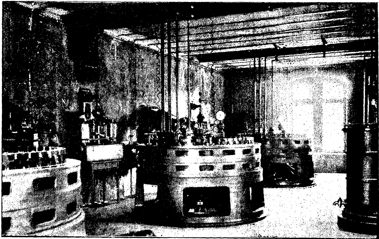
Фиг. 47. Трехфазные генераторы на центральной станции в Готцфельде.
