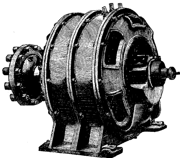
120 сильный трехфазный двигатель Бруна.
