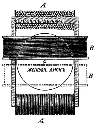
Двигатель Бореля.
