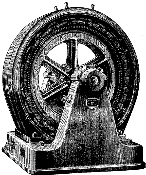
100-сильный тихоходный двухфазный двигатель Броуна.
