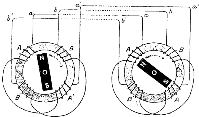
Схема двухфазной передачи энергии.
