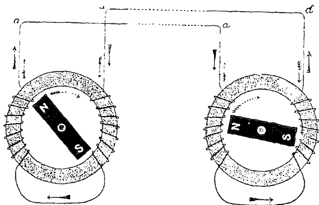
Передача энергіи отъ простаго однофазнаго альтернатора къ простаго синхронному двигателю.
