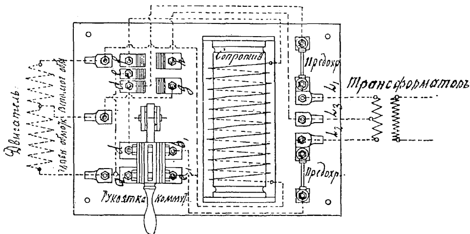
Приборъ Кольбена для пуска однофазныхъ двигателей.
