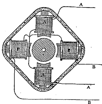
Двигатель Феррариса.
