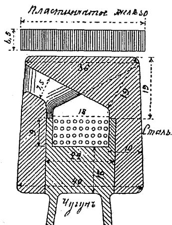
Разрѣзъ индукторовъ.
