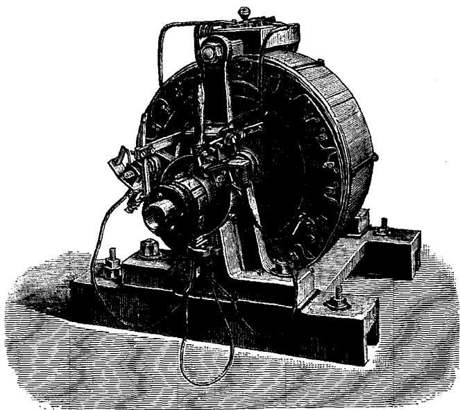
Двигатель Газельвандера (1887).
