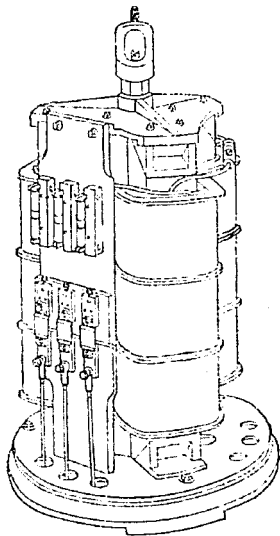
Трехфазный трансформаторъ Сименсъ и Гальске.
