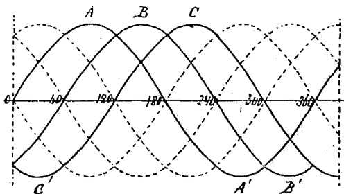
Трехфазные токи, разняшіеся по фазѣ на 60^\circ .
