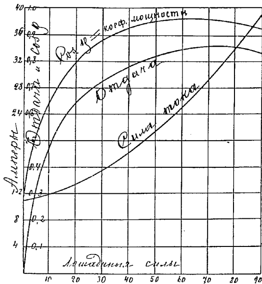
Синхронный двигатель.
