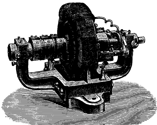
Двигатель Керпера.
