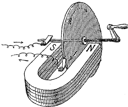
Дискъ Фарадея.
