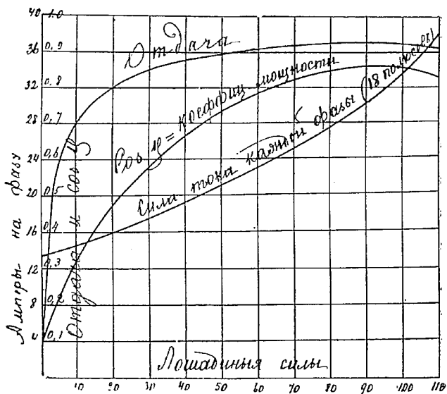
Трехфазный двигатель.
