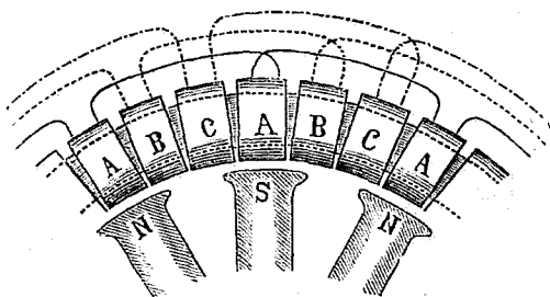
Трехфазный генераторъ.
